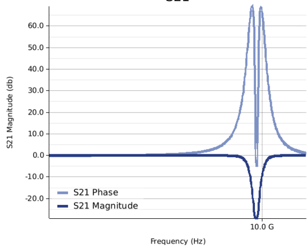
S21
